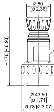
Stecker 3-polig
